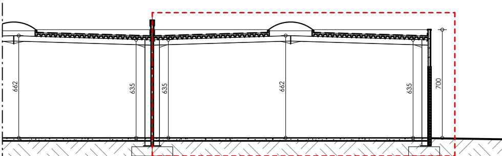
snede 1/250
