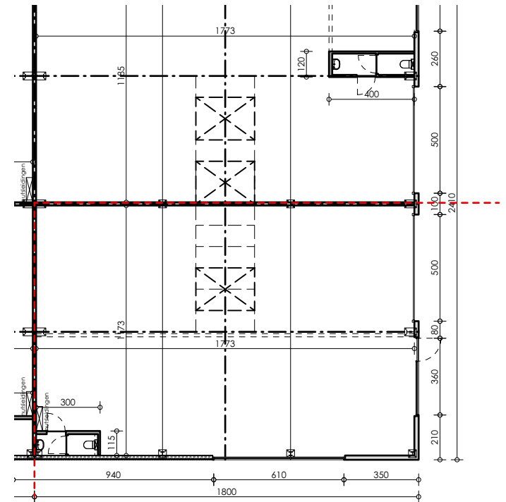
grondplan 1/250
